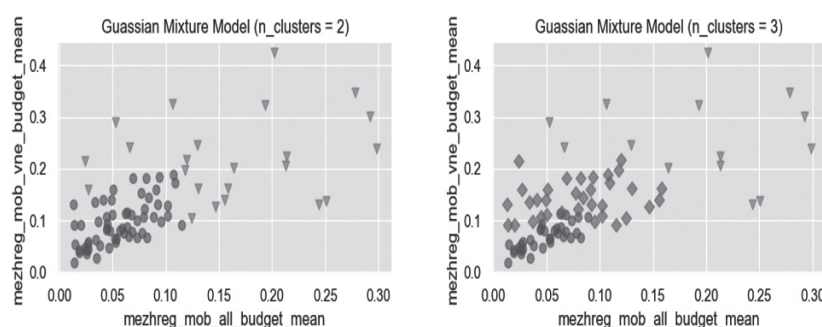
Рис. 1. Распределение 2-3 кластеров модели гауссовой смеси ( GMM ) по двум параметрам (коэффициенты межрегиональной мобильности студентов бюджетной и внебюджетной формы обучения)
